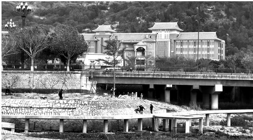
工人正在进行临水护堤挡土墙及护栏施工。
