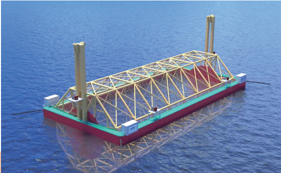
“海上牧场”效果图
