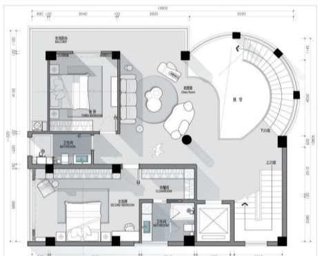
二楼平面方案
