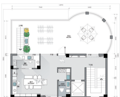
四楼平面方案
